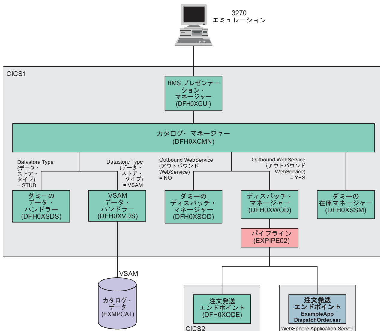
図 30. ベース・アプリケーションの構造
