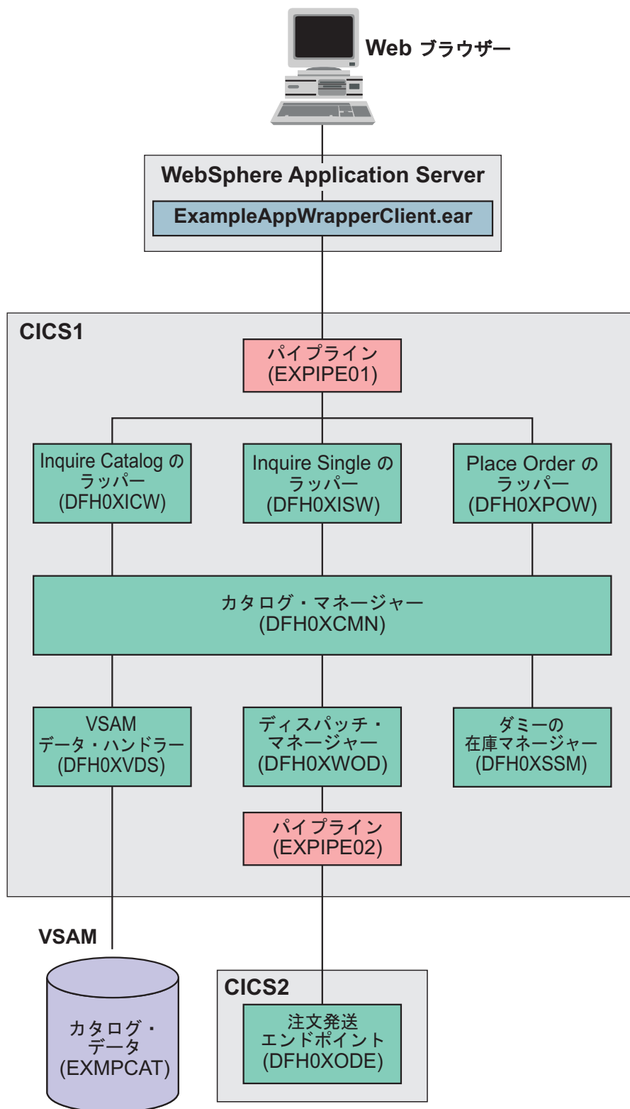
図 32. 代替の Web サービス・プロバイダー構成
