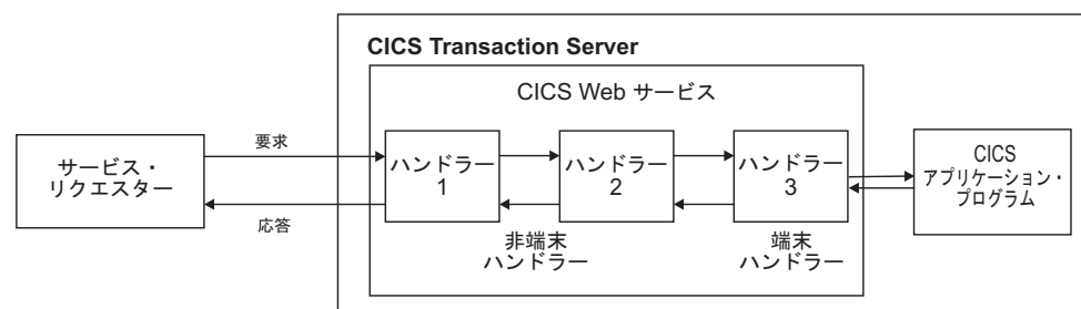
図 23. サービス・プロバイダー・パイプラインでのハンドラーの順序
