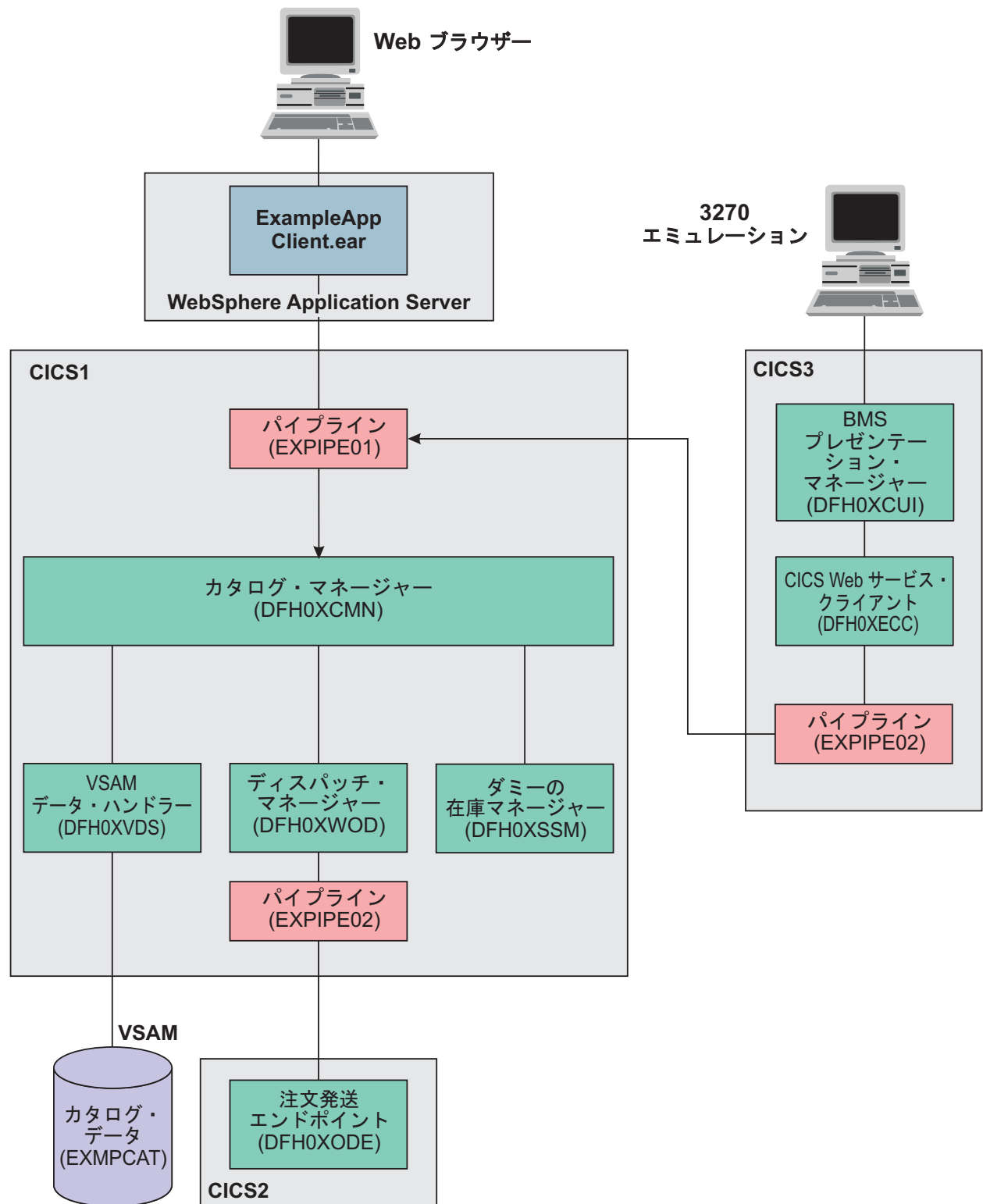
図 31. Web サービス・プロバイダーとして構成された実例アプリケーション
