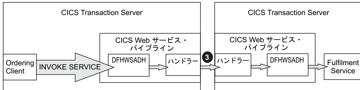
図 29. Ordering Client から Fulfilment Service への要求
