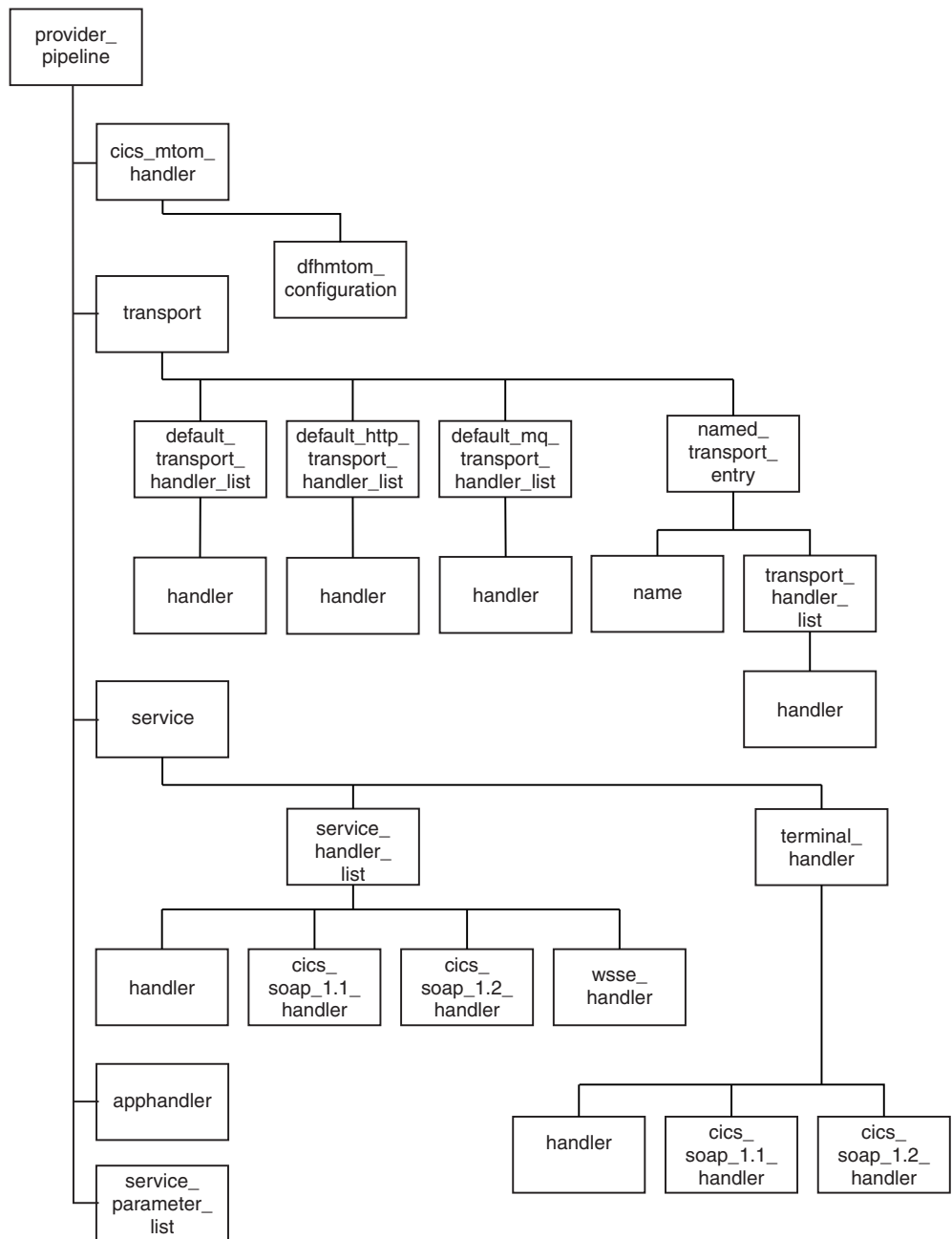
図 21. サービス・プロバイダーのパイプライン定義の構造：
