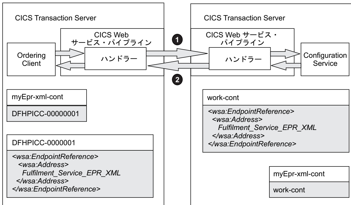
図 28. Ordering Client と Configuration Service の間の要求/応答メッセージの交換
